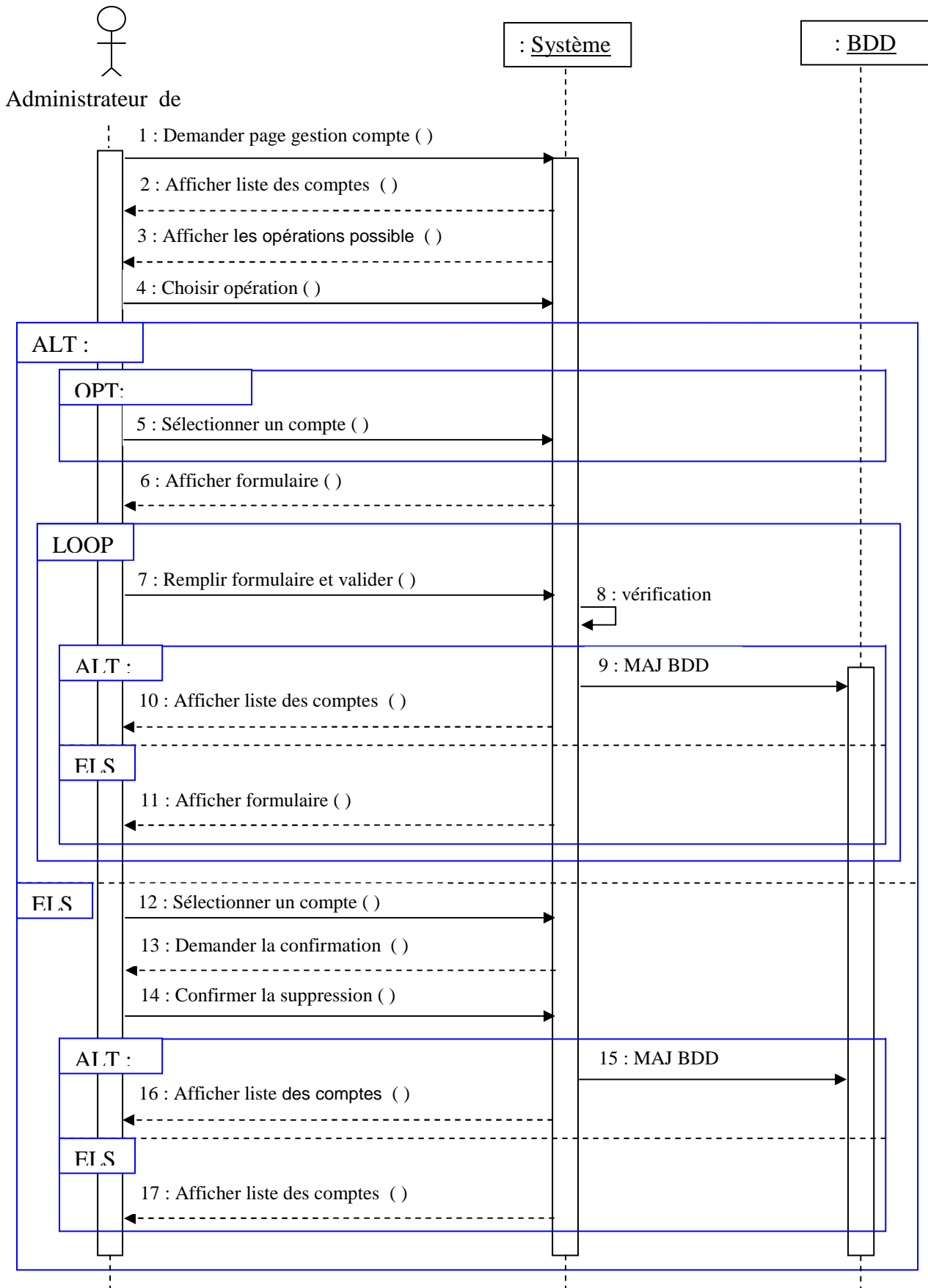
Figure 2.2.29 : Diagramme de séquence « Gérer compte »
