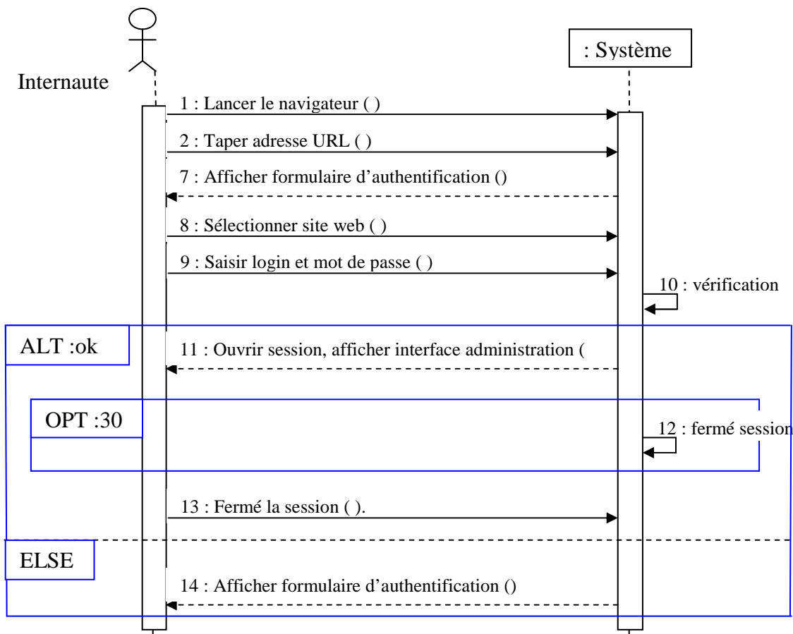
Figure 2.2.19 : Diagramme de séquence « Authentification »
