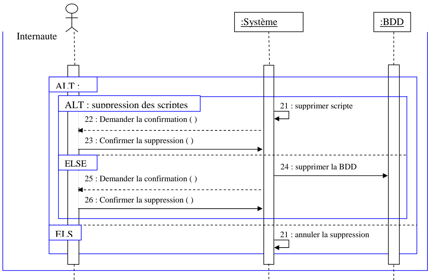
Figure 2.2.26 : Diagramme de séquence « Crée site »
