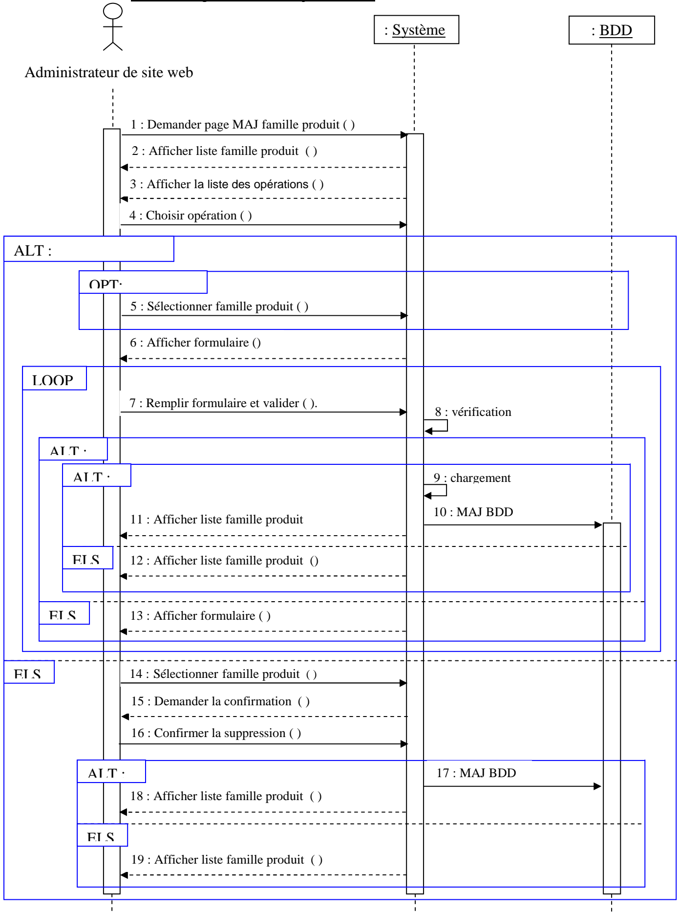
Figure 2.2.22 : Diagramme de séquence « Mettre a jour famille
