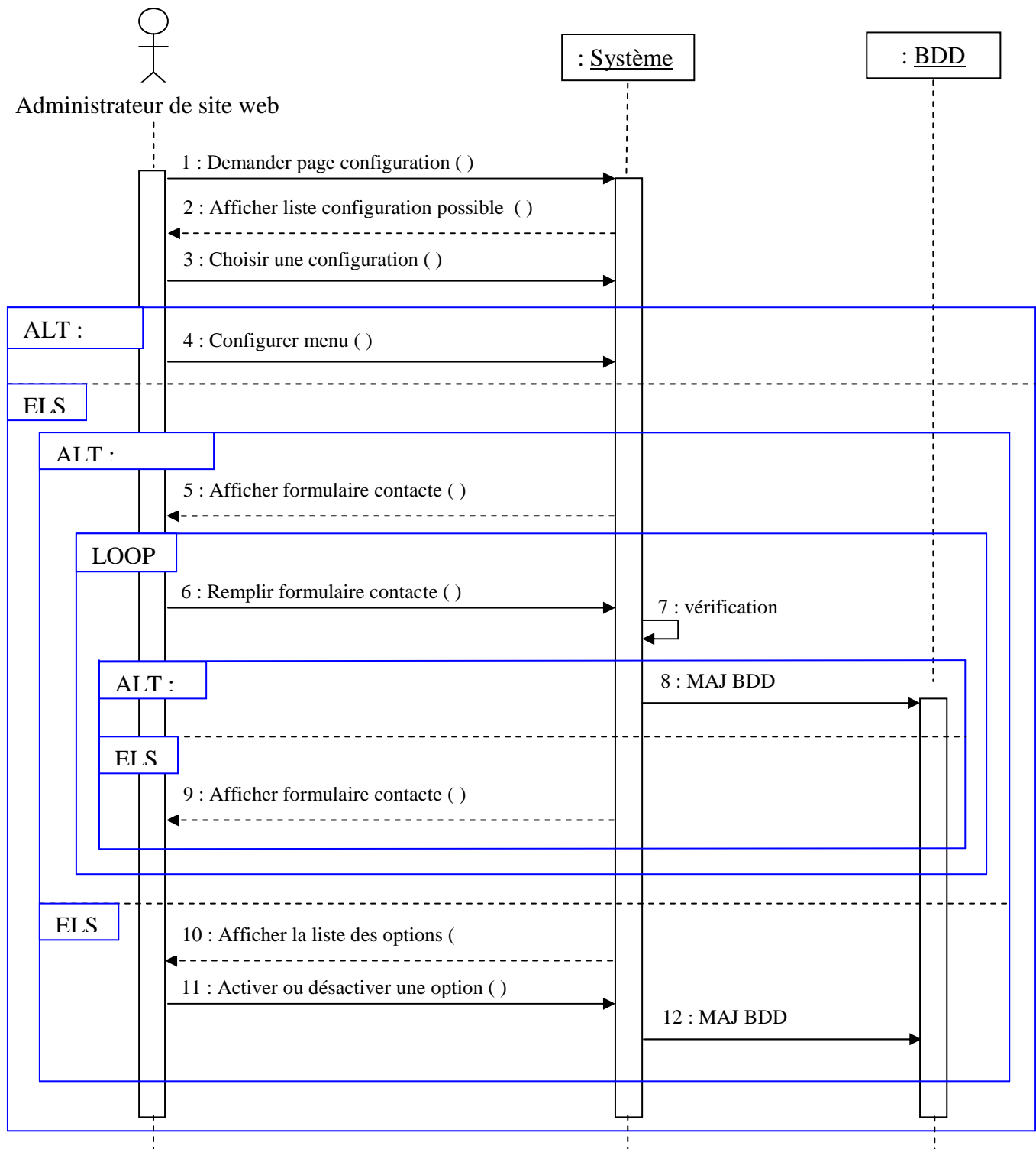
Figure 2.2.27 : Diagramme de séquence « Configurer site »
