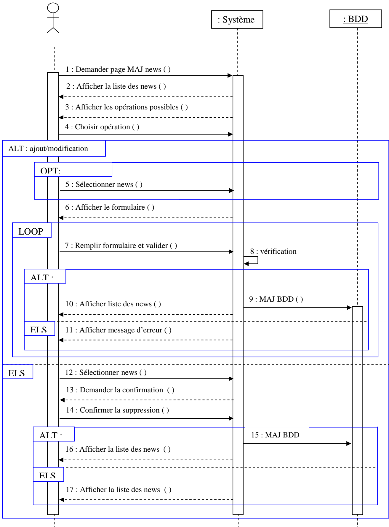
Figure 2.2.21 : Diagramme de séquence « Mettre a jour news »
