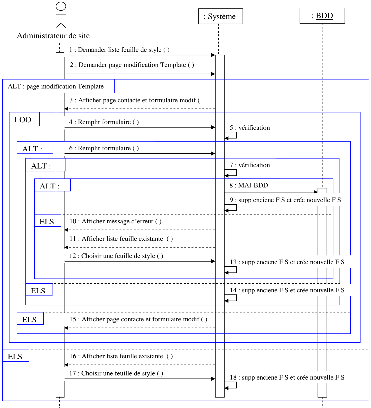
Figure 2.2.24 : Diagramme de séquence « Modifier Template »
