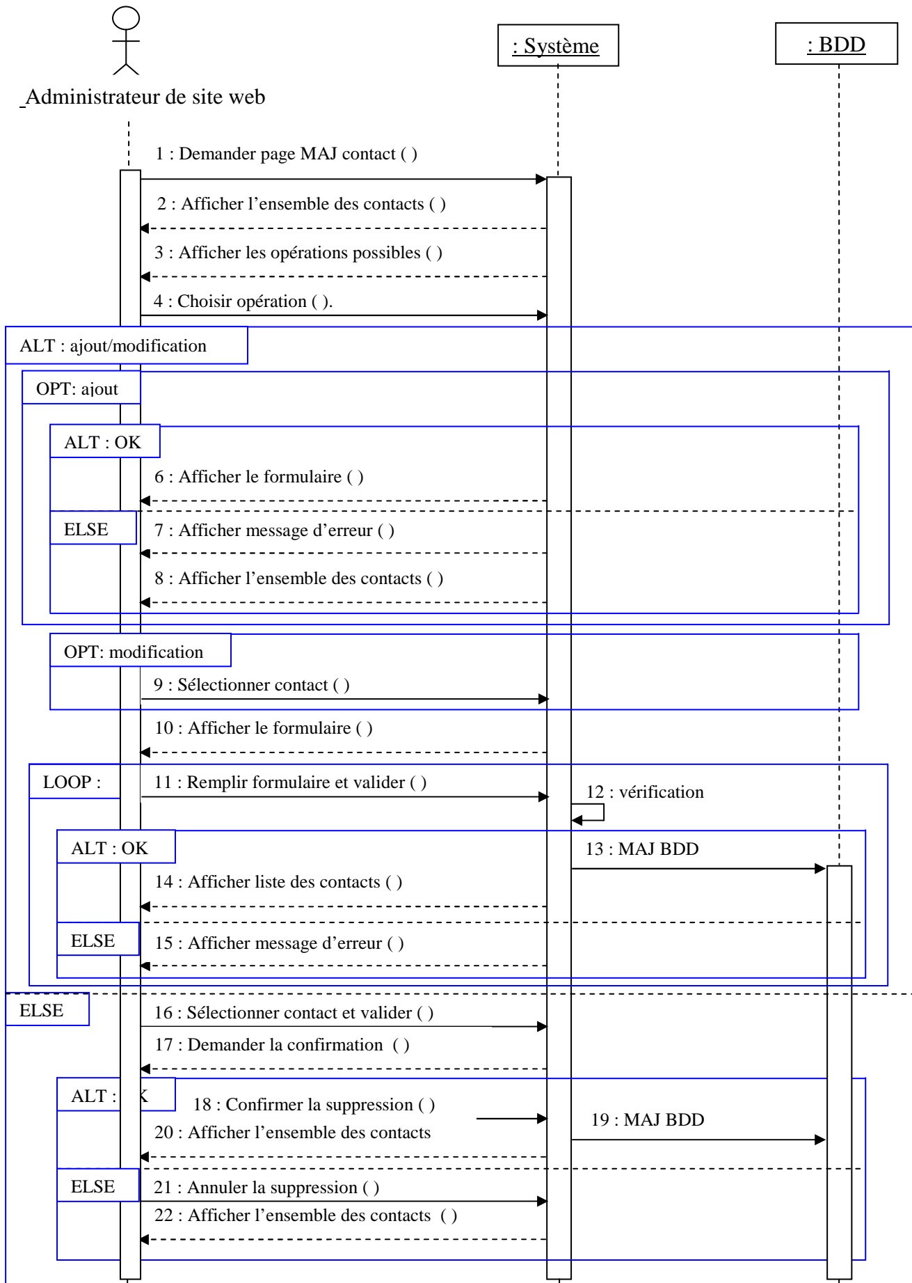
Figure 2.2.30 : Diagramme de séquence « Mettre à jour contact »
