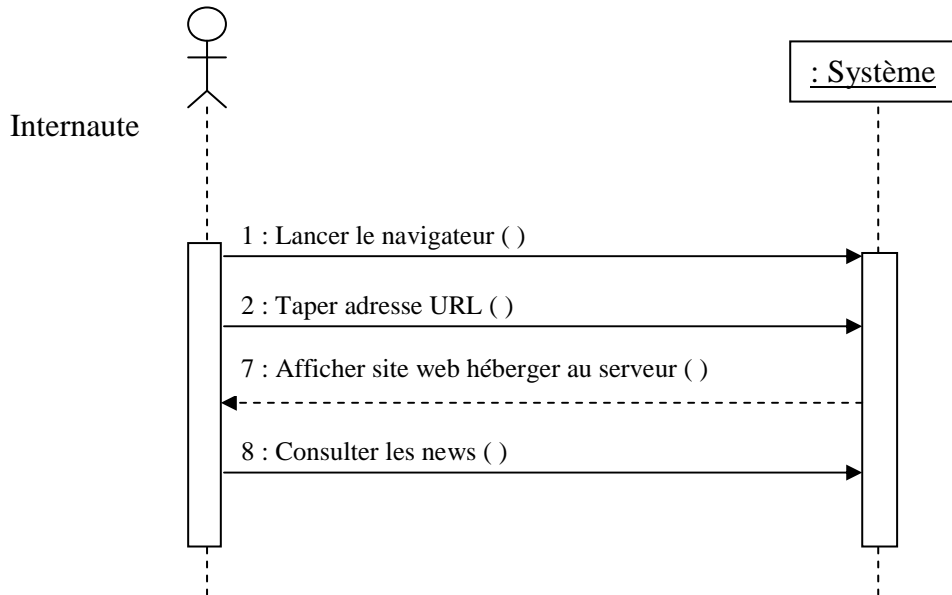
Figure 2.2.16 : Diagramme de séquence « Consulter NEWS »
