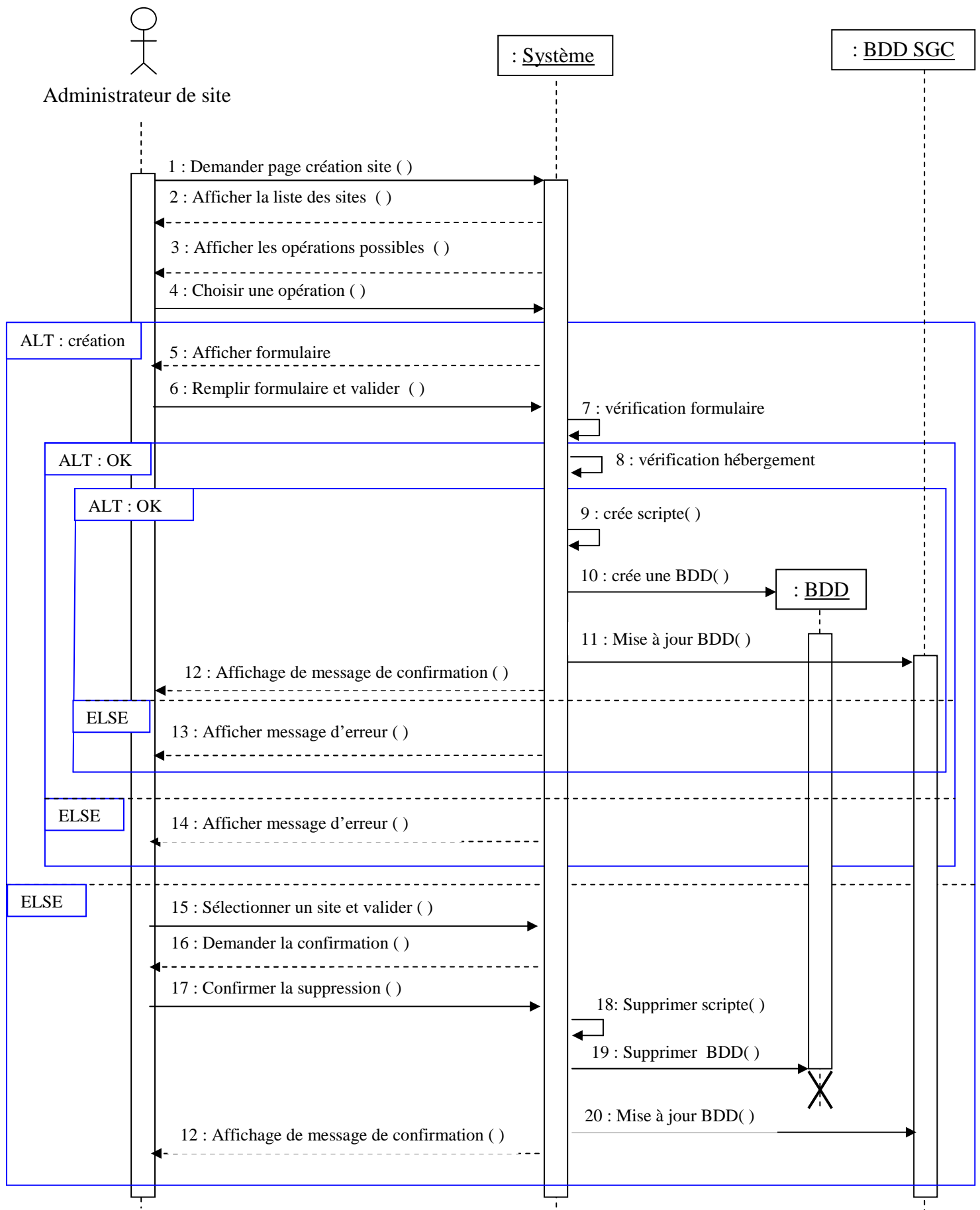
Figure 2.2.26 : Diagramme de séquence « Crée site »
