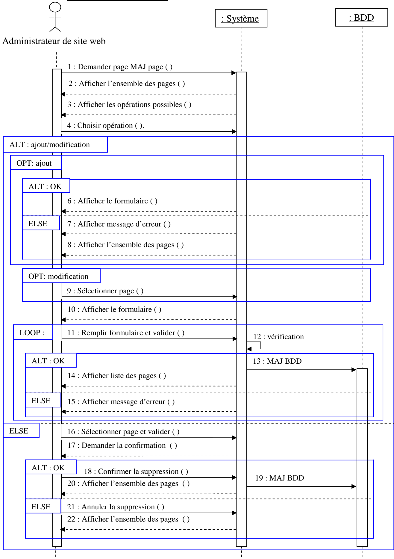
Figure 2.2.23 : Diagramme de séquence « Mettre a jour page »
