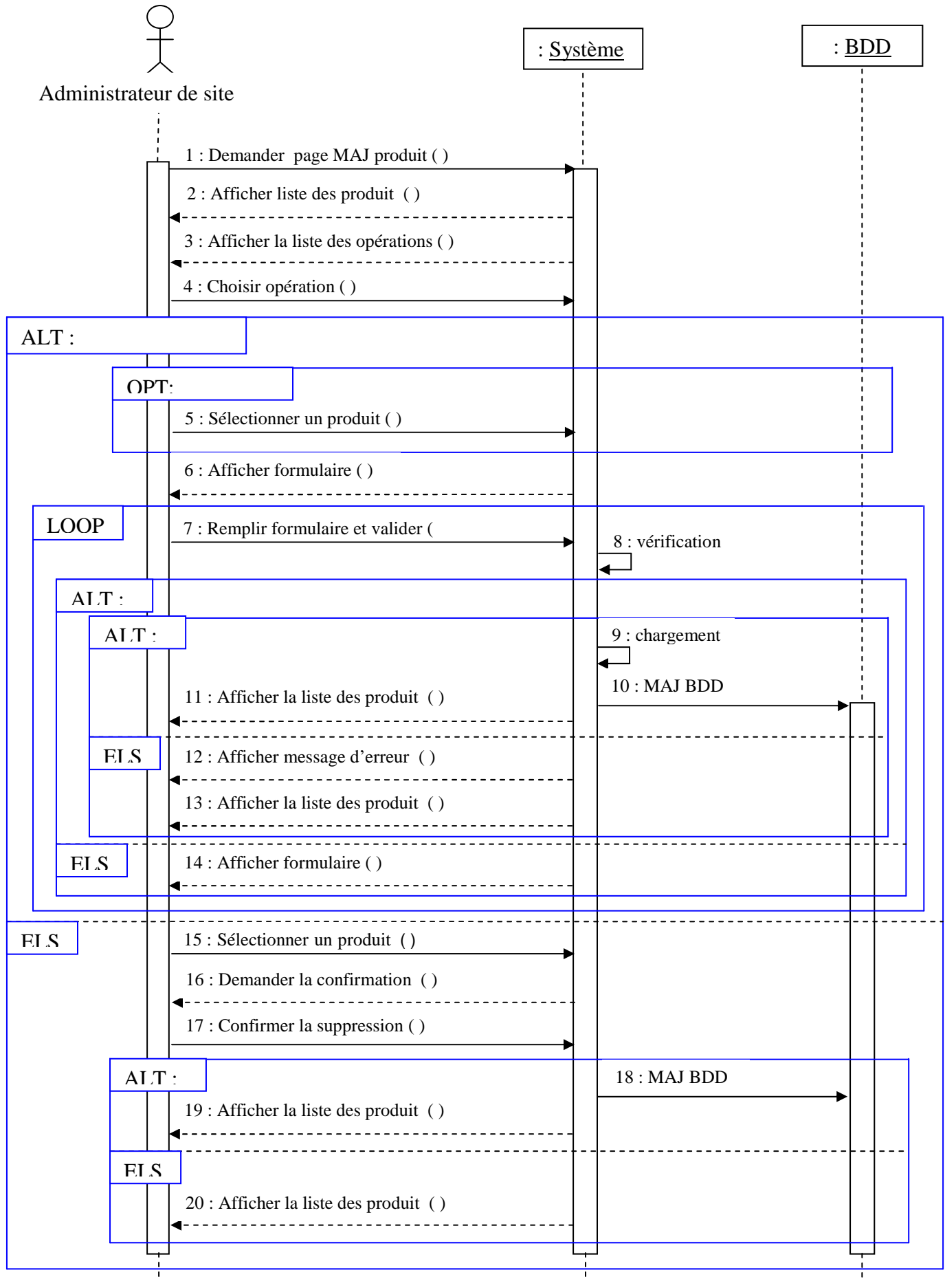
Figure 2.2.25 : Diagramme de séquence « MAJ Catalogue produits »
