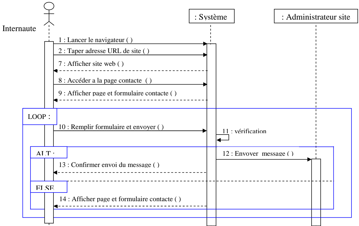
Figure 2.2.18 : Diagramme de séquence « Envoyer message »
