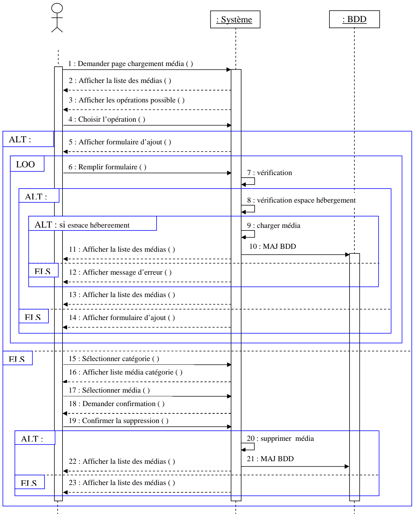
Figure 2.2.20 : Diagramme de séquence « Charger média »
