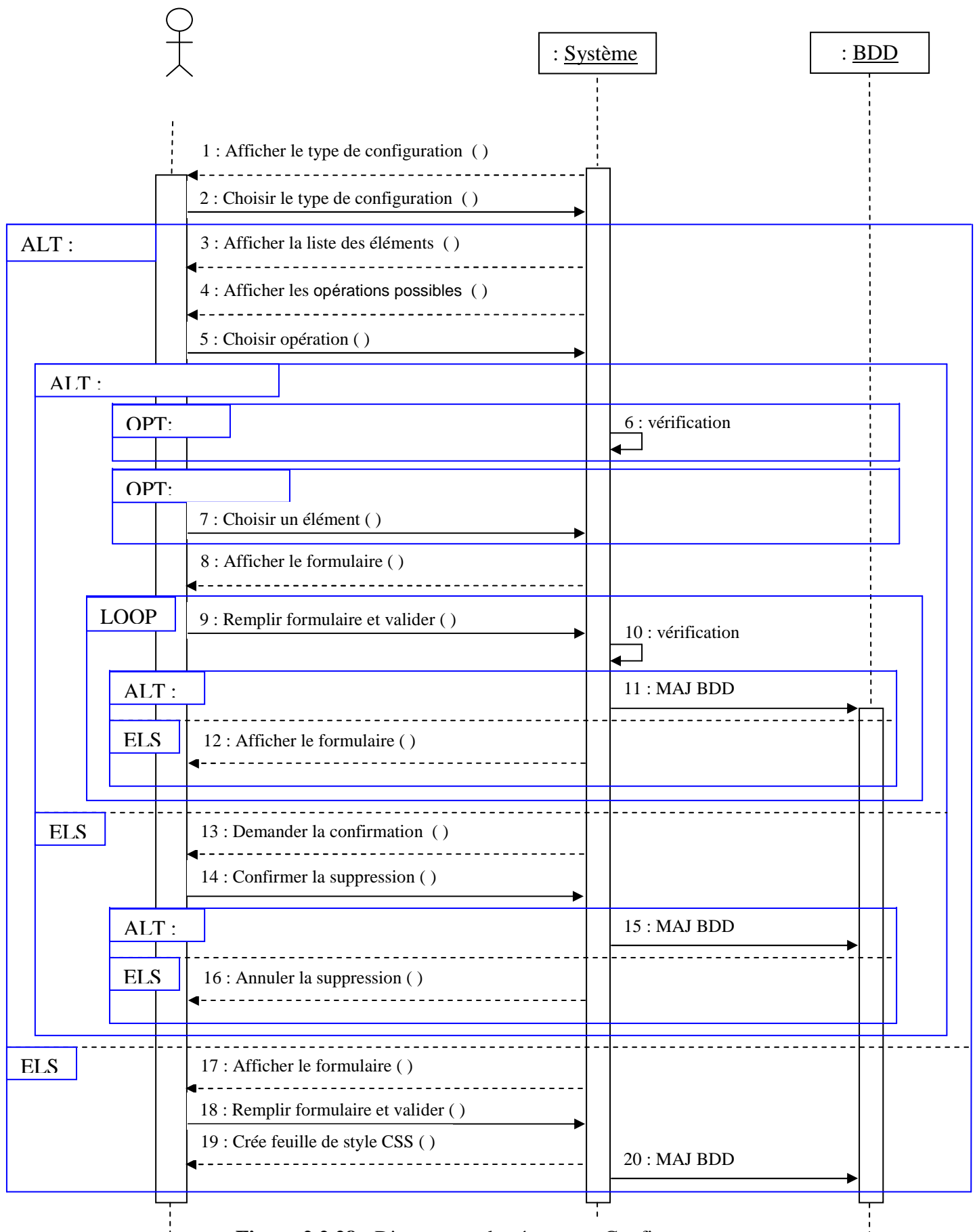
Figure 2.2.28 : Diagramme de séquence «Configurer menu »
