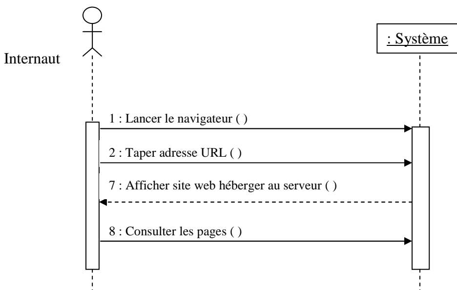
Figure 2.2.17 : Diagramme de séquence « Consulter page »
